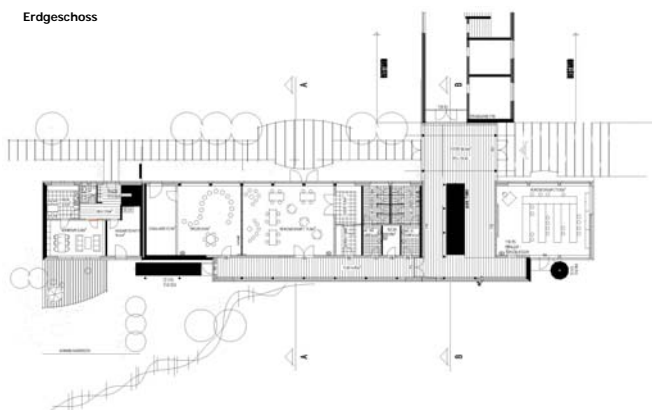
Erdgeschoss
